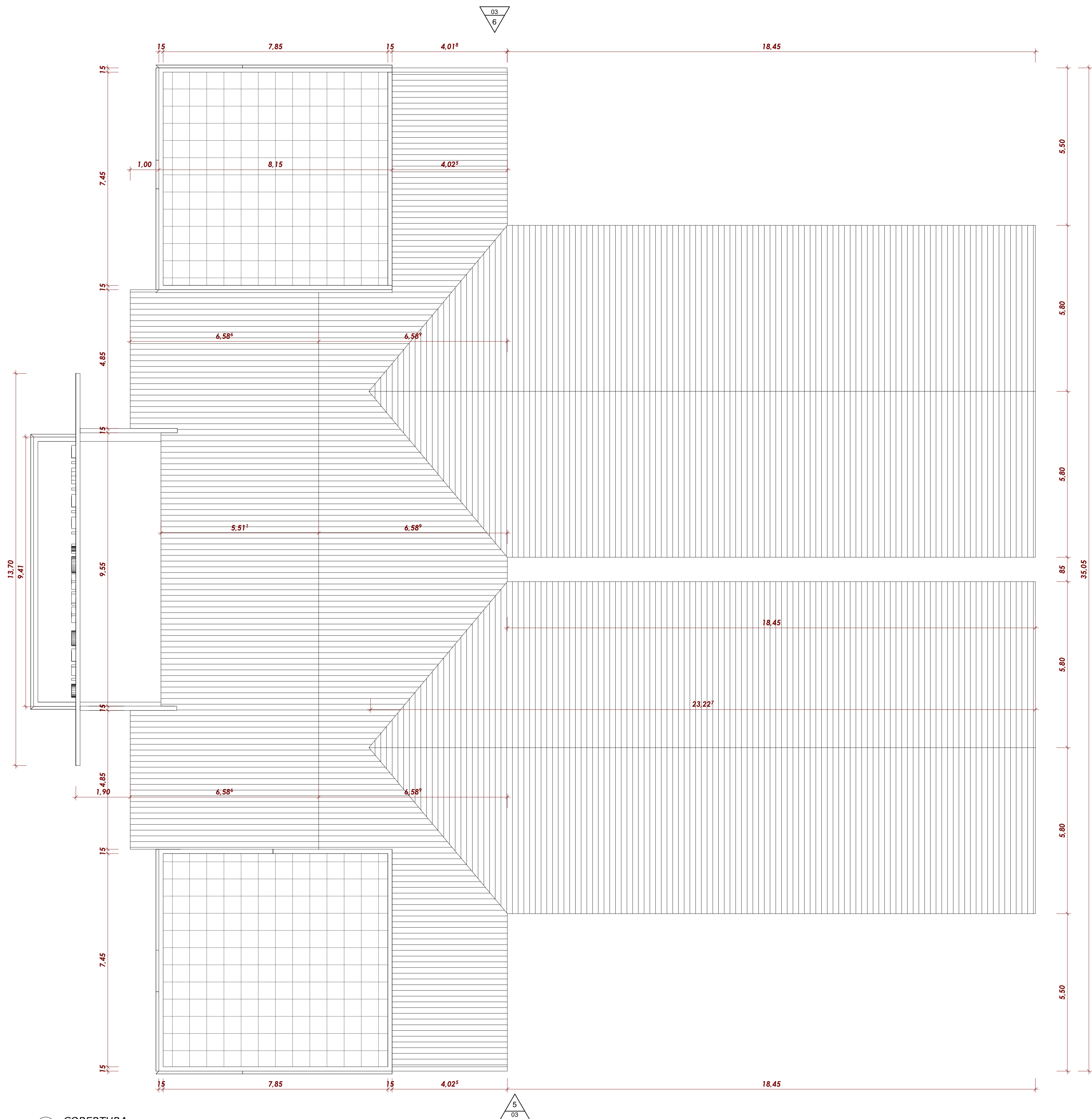
2 COBERTURA 1 : 75
