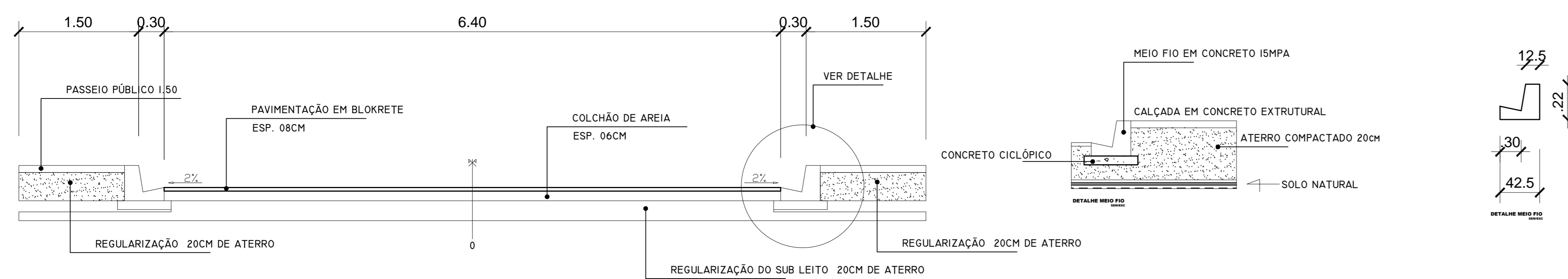
SEÇÃO TRANSVERSAL TÍPICA Esc. 1:50
